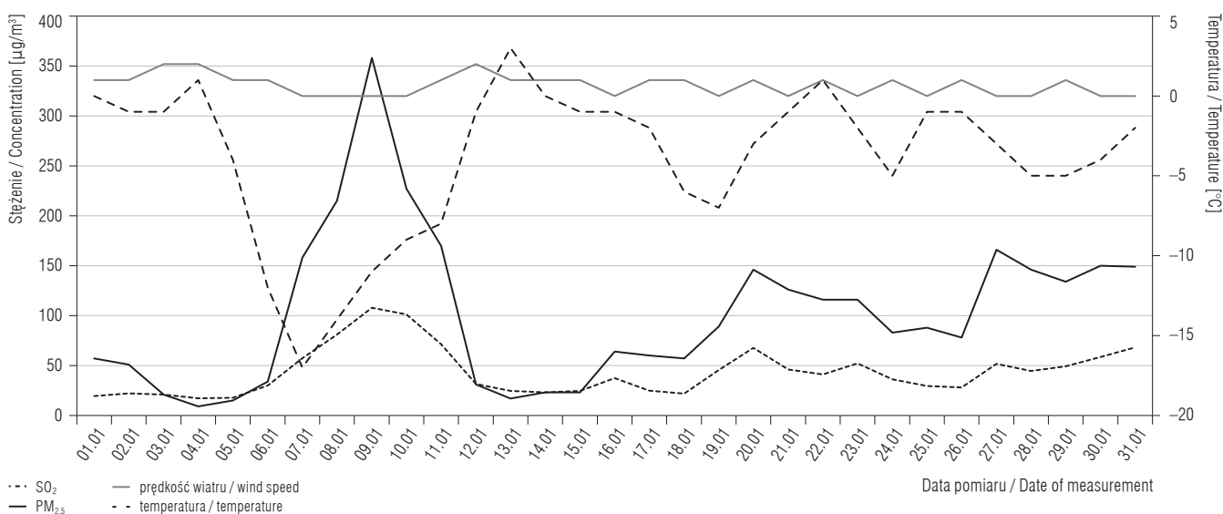
Rycina 2. Średniobowe stężenia PM 2,5 i SO 2 w powietrzu atmosferycznym oraz wybrane parametry meteorologiczne w styczniu 2017 r., wartości uśrednione dla Gliwice i Katowice
