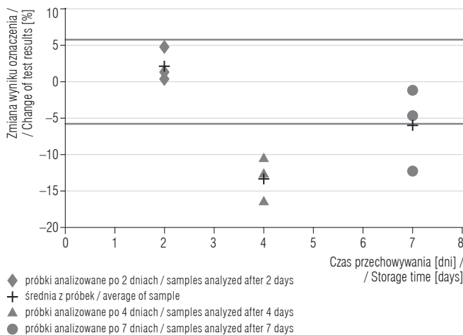
Ryc. 3. Badanie trwałości próbek 1,2:3,4-diepoksybutanu przechowywanych w chłodziarce Fig. 3. Stability test of 1,2:3,4-diepoxybutane samples stored in the refrigerator
