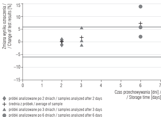
Ryc. 4. Badanie trwałości próbek 1,2:3,4-diepoksybutanu przechowywanych w zamrażarce Fig. 4. Stability test of 1,2:3,4-diepoxybutane samples stored in the freezer
